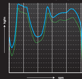
軸トルク曲線図 FW Torque Graph
